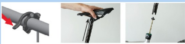
Figur 112: Udtrækning af sadelpind
