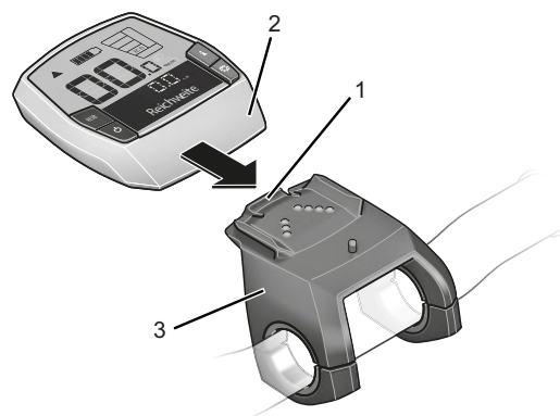
Figur 72: Skub cykelcomputeren (2) hen over cykelcomputerens lås (1) indtil anslag i holderen (3)
