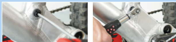
Figur 141: Fastgørelse af postpin-aksel
